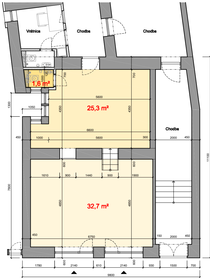
Pôdorys predajne
